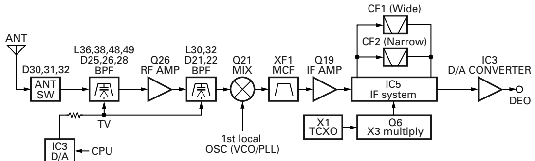
Fig. 2 Receiver system / 图2 接收部系统
